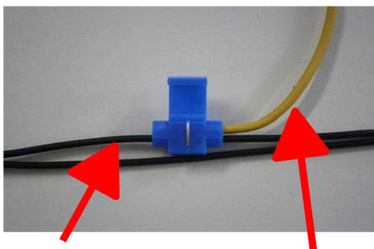
DC- Minusleitung
